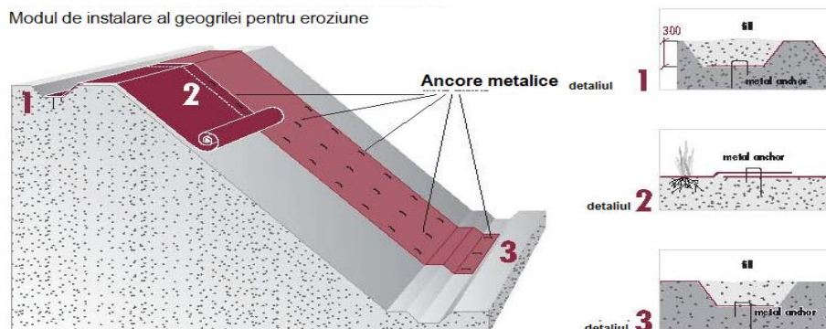
Modul de instalare al geogrilei pentru eroziune
